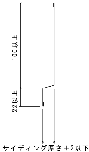
<タイプA> 役物(中間水切り)の形状
