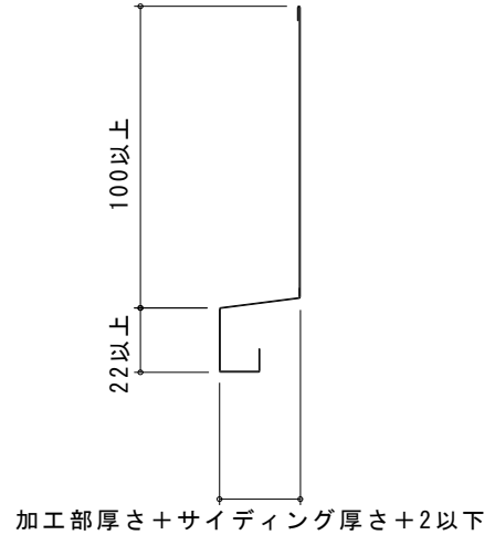
<タイプB> 役物(中間水切り)の形状
